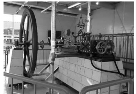
製糸場に展示されているブリュナエンジン
