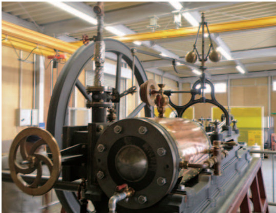
富岡商工会議所工業部会によって 復元されたブリュナエンジン
